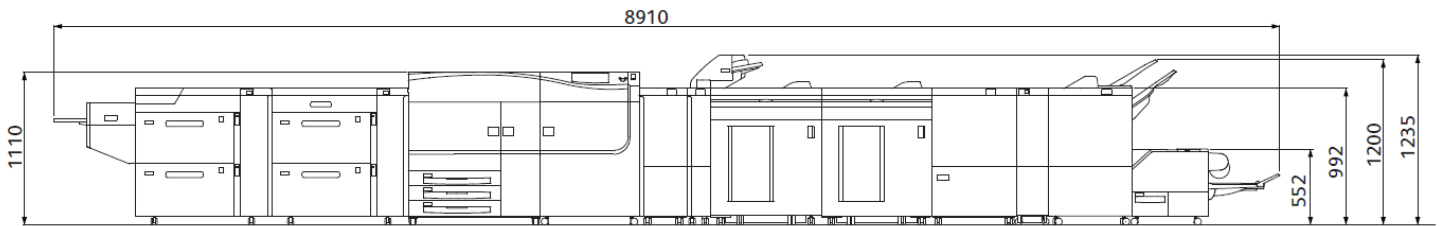
正面図
