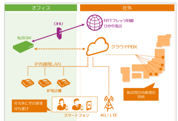
システム構成図
